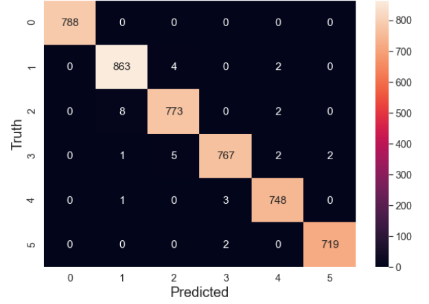
Fig. 7. RFC confusion matrix.
