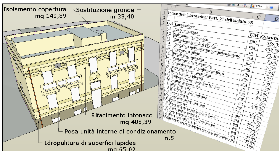
Figura 2. Reggio Calabria. Isolato 78. Computo Metrico Grafico (Massimo, 2009)
