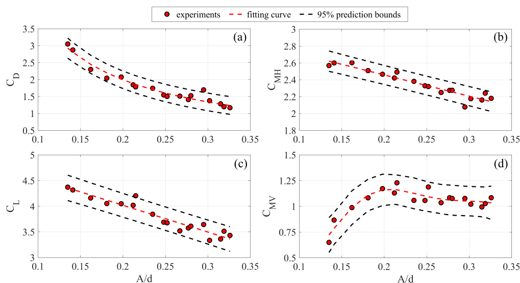
Figure 11. Hydrodynamic coefficients vs. A/d . (a) C_D ; (b) C_{MH} ; (c) C_L ; (d) C_{MV} .
